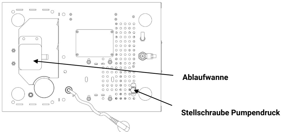
Abb. 5 Unterseite Maschine
